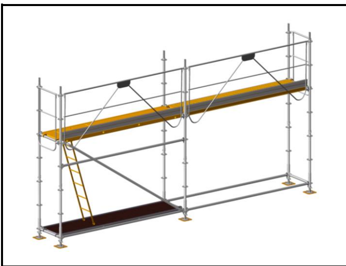
9 Placez puis verrouillez les planchers à l'aide des anti-soulèvements, puis insérez les crochets de l'échelle autour de l'échelon sous le plancher trappe. Enfin, enlevez le plancher sur lequel l'échelle ne repose pas
