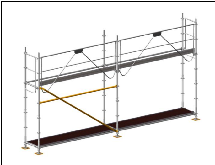
8 Positionnez puis clavetez la diagonale ainsi qu'un longeron à 1,5 m afin de sécuriser l'accès à l'échelle.
