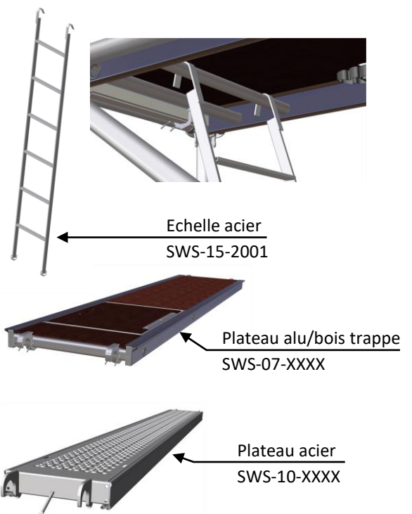
9 Placez puis verrouillez les planchers à l'aide des anti-soulèvements, puis insérez les crochets de l'échelle autour de l'échelon sous le plancher trappe. Enfin, enlevez le plancher sur lequel l'échelle ne repose pas
