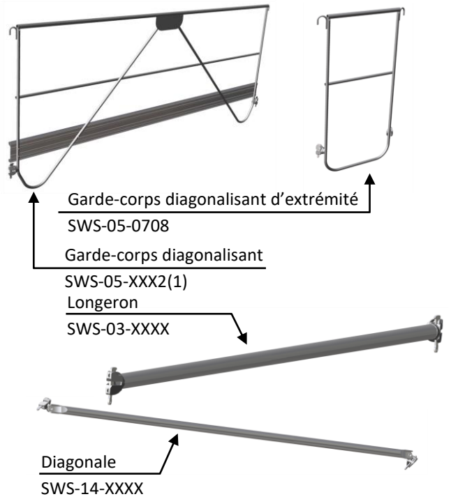
7 Positionnez et clavetez les garde-corps diagonalisant de l'étage supérieur.
