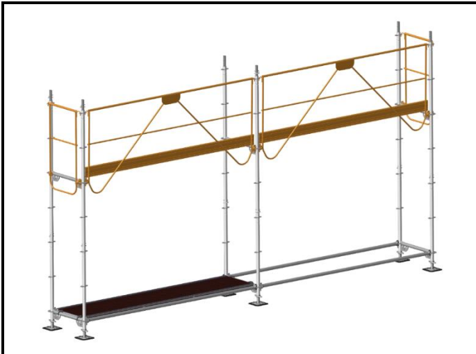
7 Positionnez et clavetez les garde-corps diagonalisant de l'étage supérieur.
